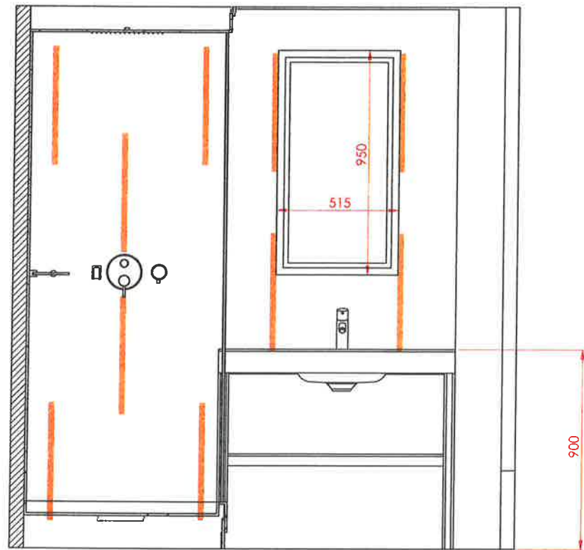
COUPE B-B ECHELLE 1 : 12
