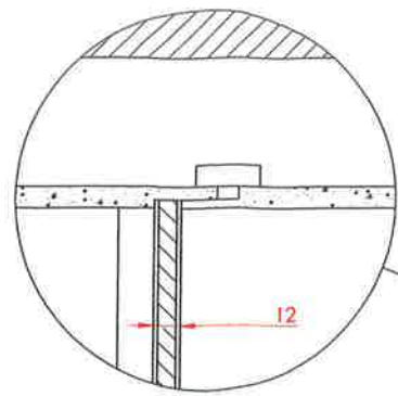
DÉTAIL G ECHELLE 1 : 2
